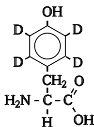
tyrosine-d 4
